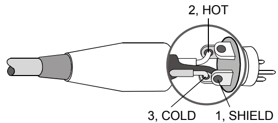
Abbildung 2-2: Symmetrische Belegung von XLR male
