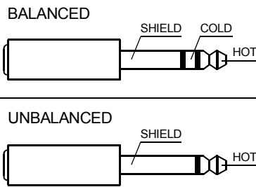
Abbildung 2-1: Symmetrische bzw. unsymmetrische Belegung des Klinkenstecker
