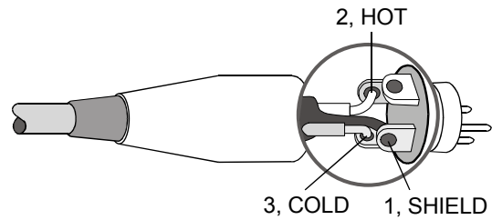
Illustration 2-2: Câbles audio symétrisés (XLR, male)
