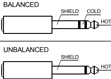
Illustration 2-1: Jack stéréo
