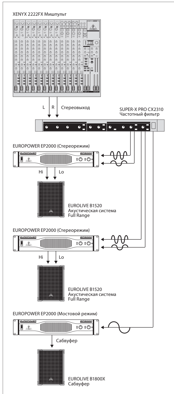
Рис. 3.7: Стереорежим Bi-Amp с отдельным сабвуфером
