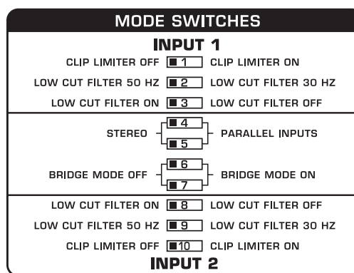
Рис. 2.3: DIP-переключатель EUROPOWER
