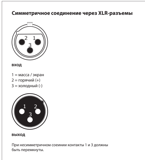
Рис. 4.3: Разъемы XLR
