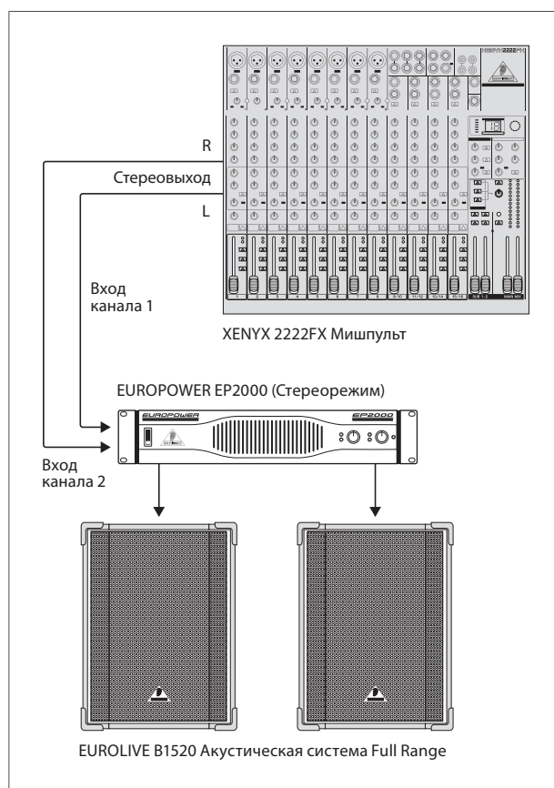
Рис. 3.1: Двухканальный режим
